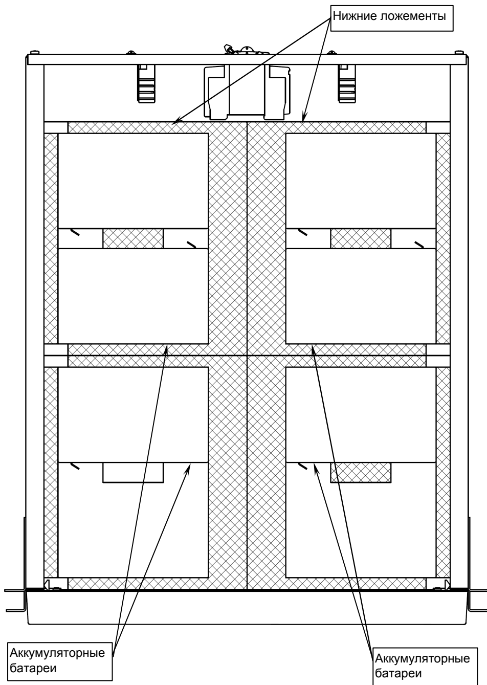
Рисунок 3 – Размещение аккумуляторных батарей в корпусе
